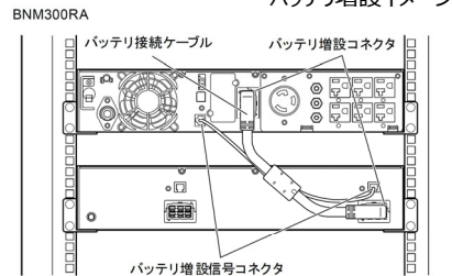
バッテリー増設イメージ
