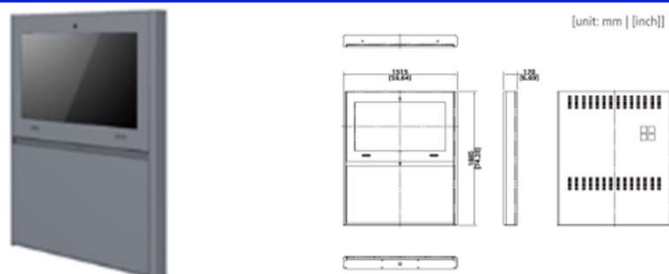
屋外用55インチ横モデル(キャスターなし)
