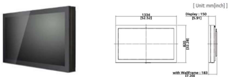
屋外用55インチ壁掛けモデル
