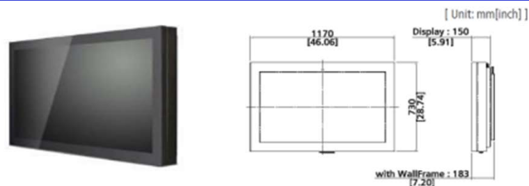
屋外用46インチ高輝度壁掛けモデル
